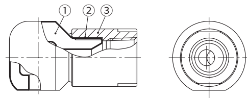
①ノズル本体 ②接着剤：アラルライト®H ③ソケット
