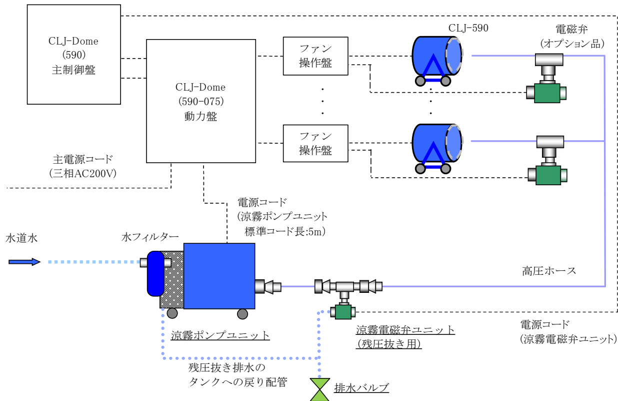
(1) CLJ-Dome 制御盤機器フロー図
