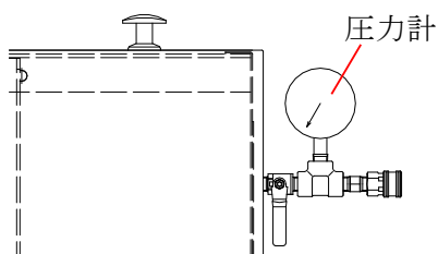
吐出部1/4(上面図)
