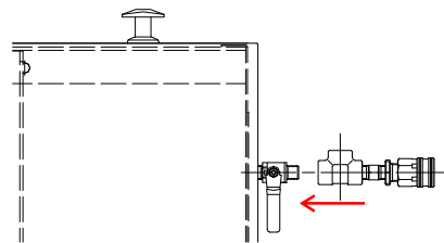
吐出部3/8(上面図)
