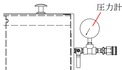
吐出部3/8(上面図)
