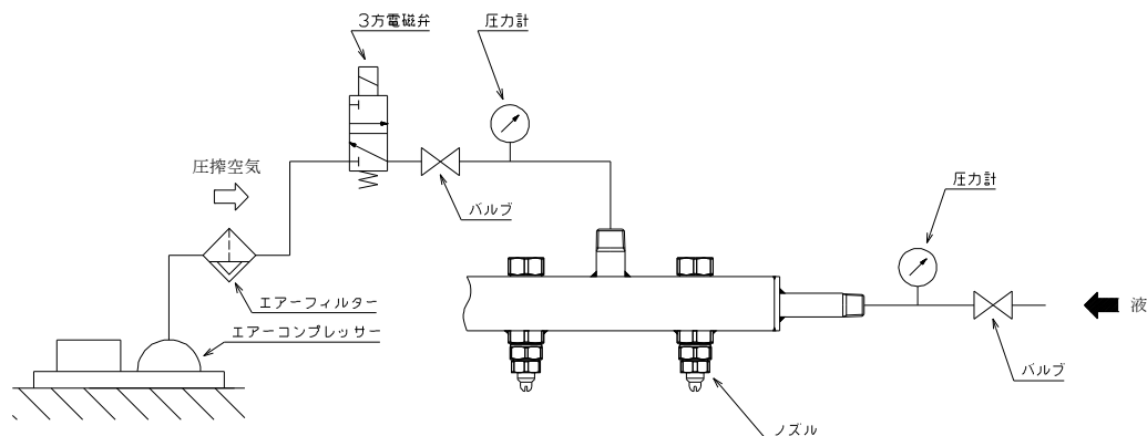
図2. 3方電磁弁を使用した配管方法例
