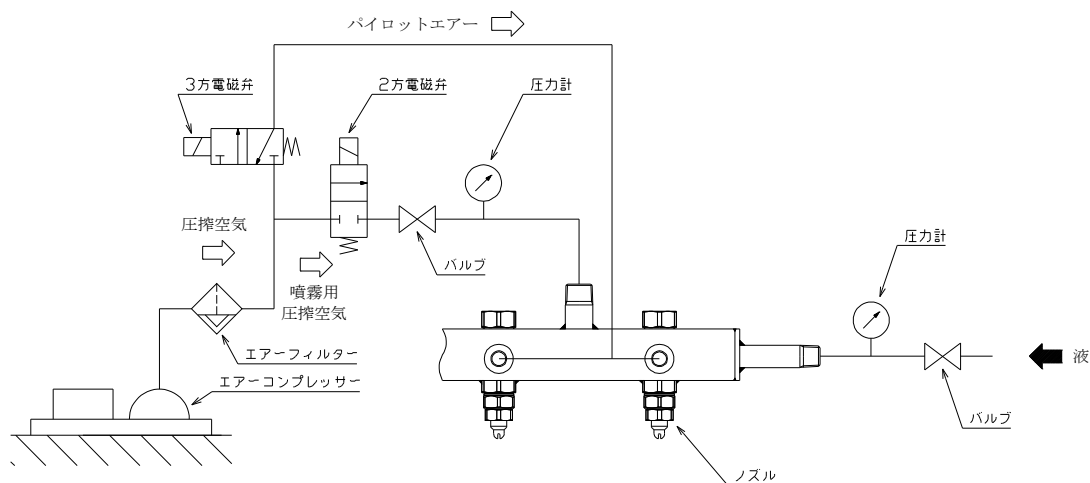
図 1. 3 方電磁弁を使用した配管方法例
