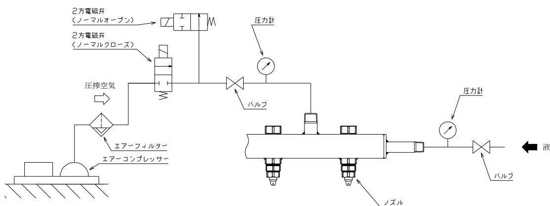
図3. 2方電磁弁を使用した配管方法例
